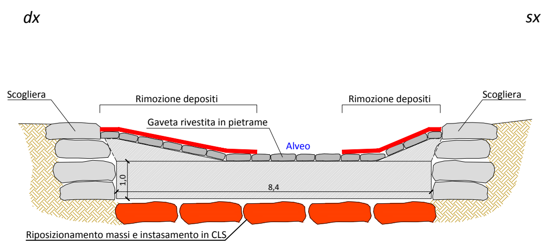
BRIGLIA 2
