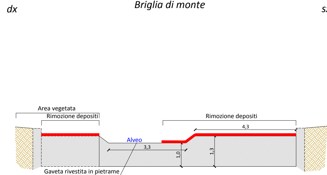
BRIGLIA 7
