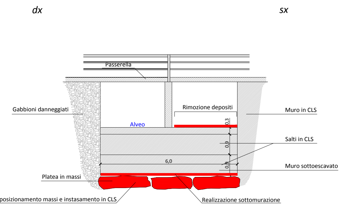
BRIGLIA 9
