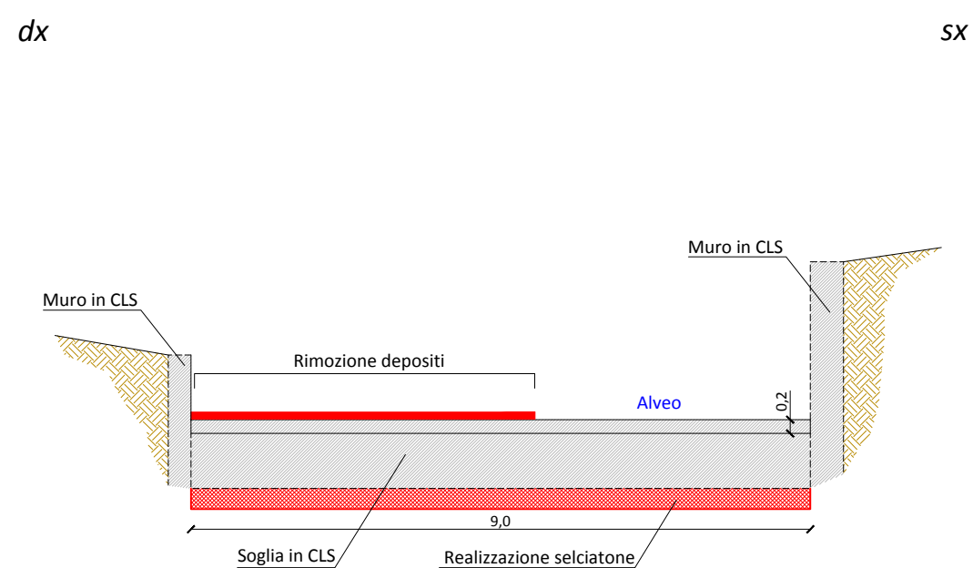
SOGLIA 5
