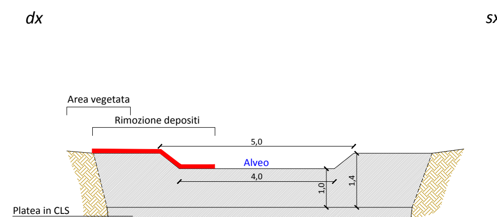
BRIGLIA 8A
