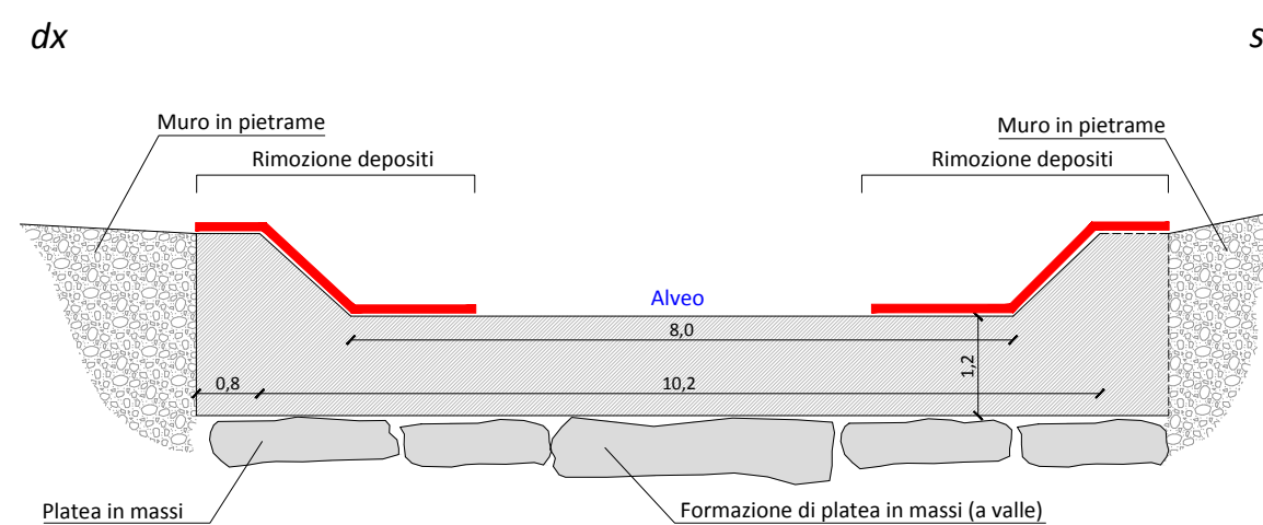
BRIGLIA 12
