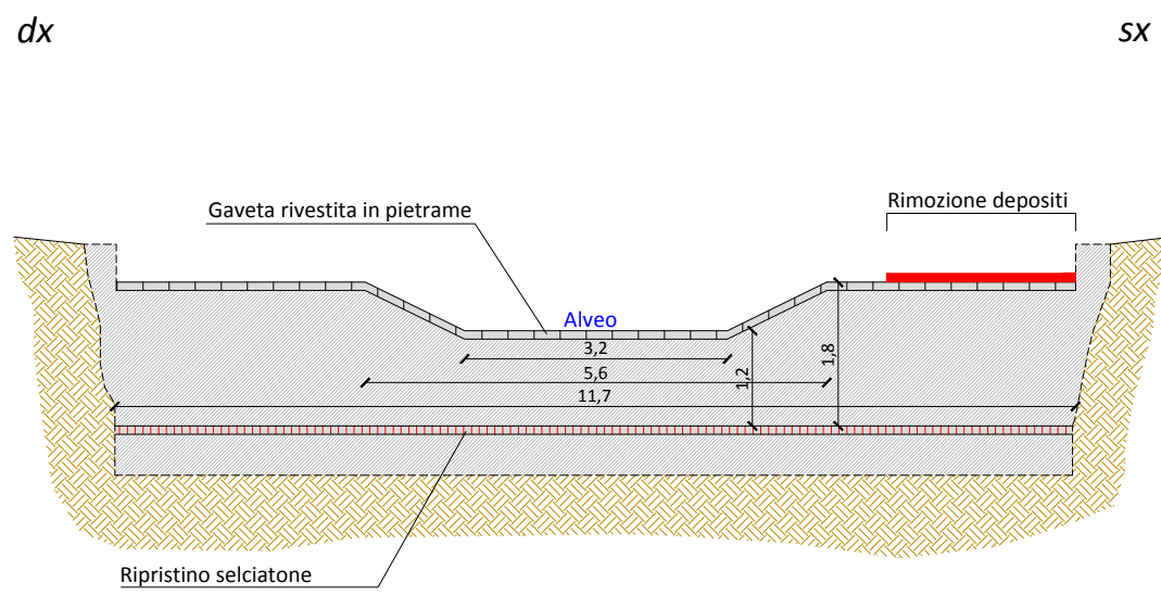
BRIGLIA 1
