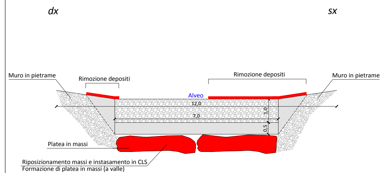
BRIGLIA 11
