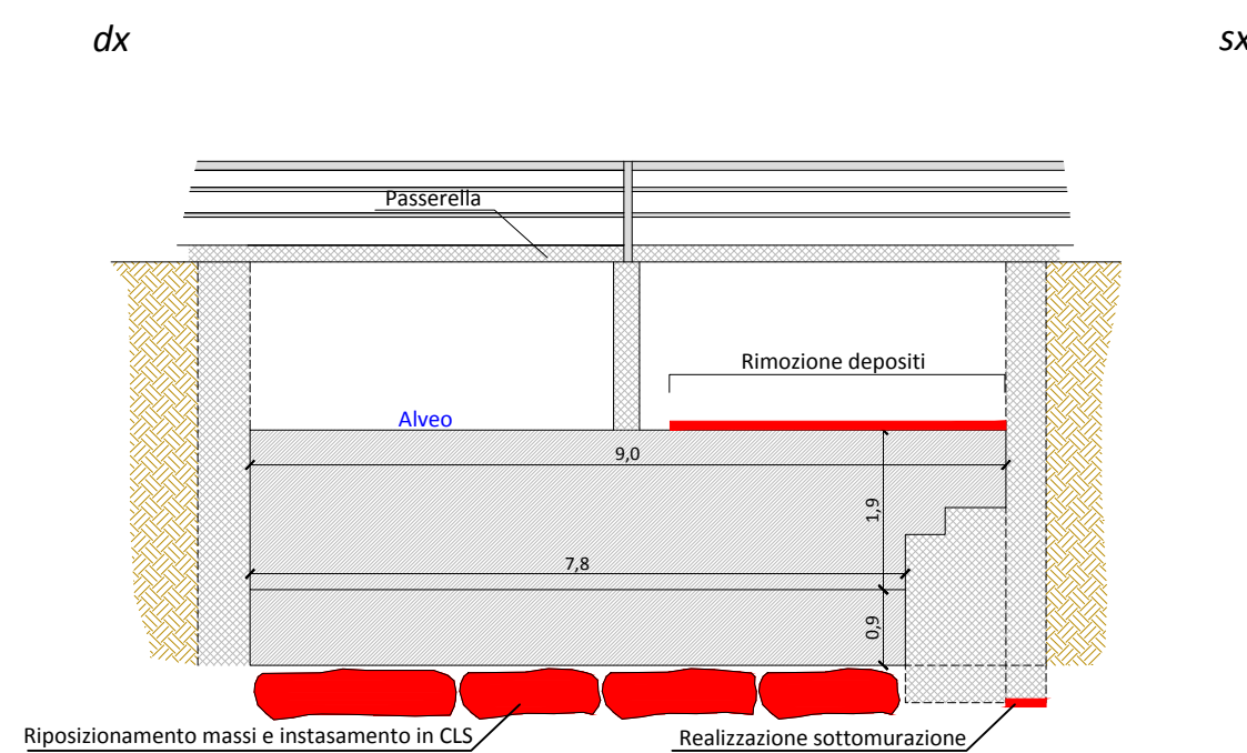
BRIGLIA 7
