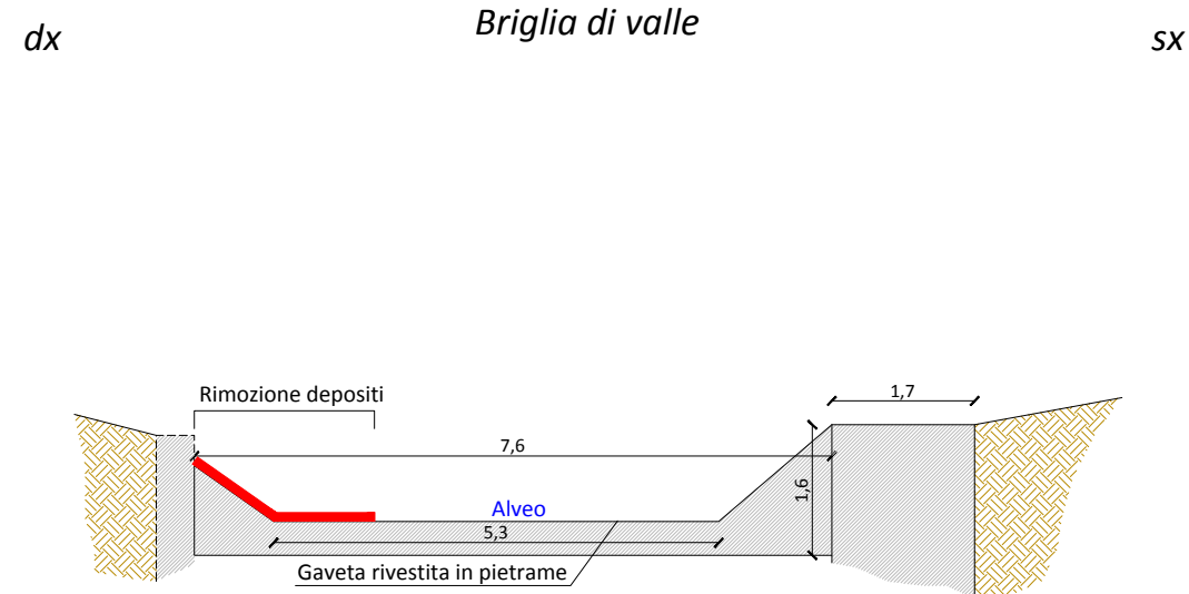
BRIGLIA 7
