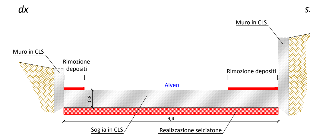
SOGLIA 4
