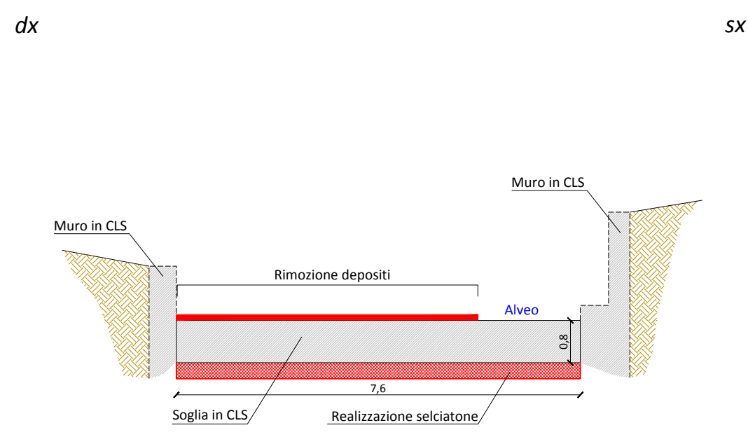
SOGLIA 6
