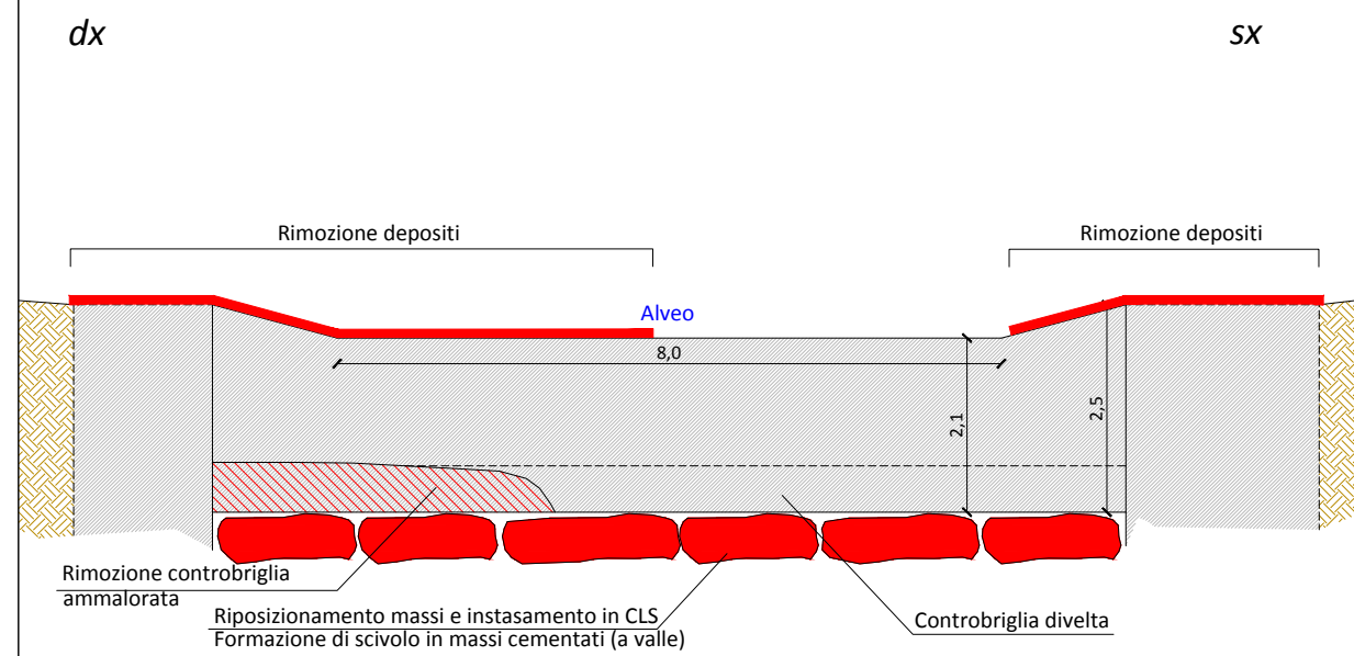
BRIGLIA 8
