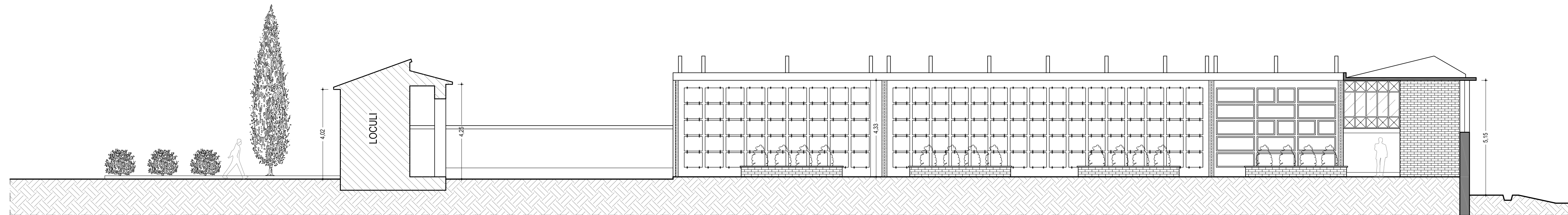
1 SEZIONE LONGITUDINALE A-A Scala: 1:100 - misure in metri
